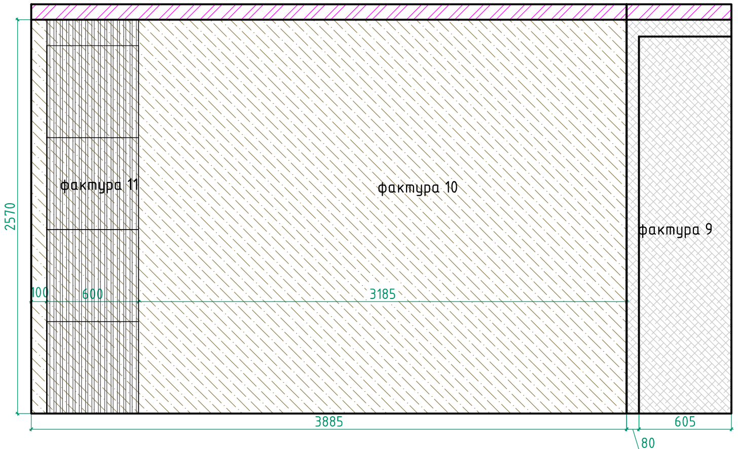
Вид Г2(кухня)
