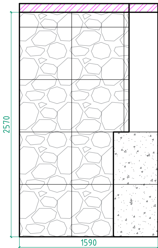
Вид Д1(Туалет)
