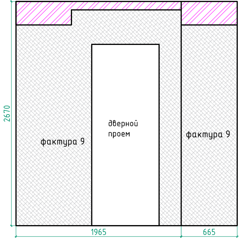
Вид Г5(кухня)
