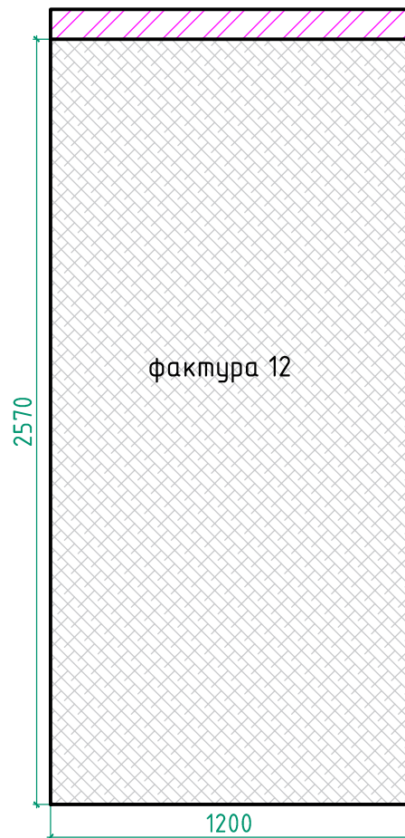
Вид E2(гардероб)
