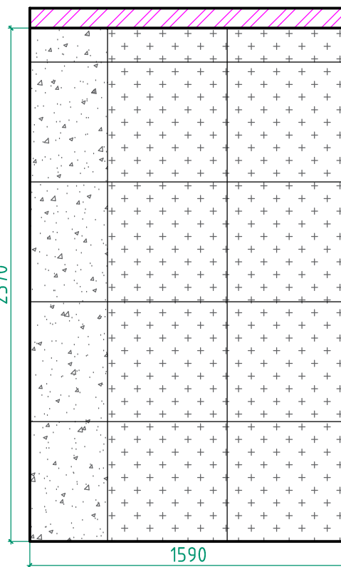
Вид Д3(Туалет)
