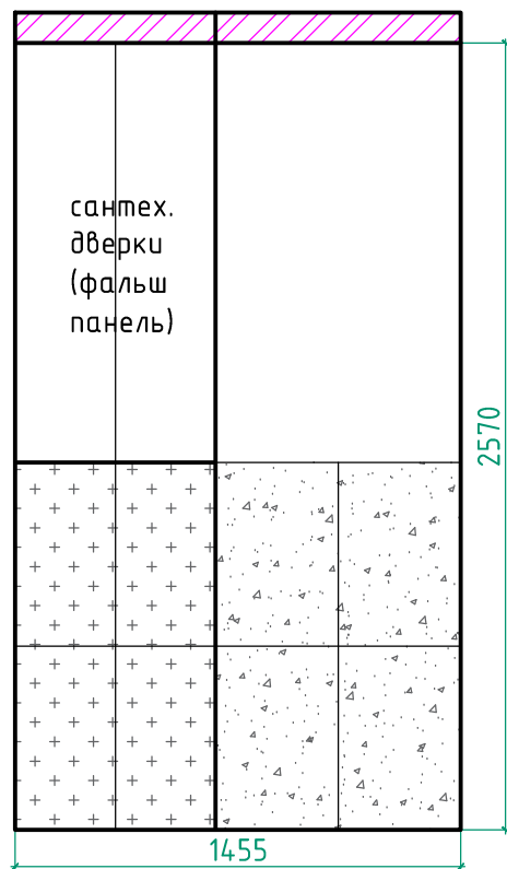
Вид Д2(Туалет)
