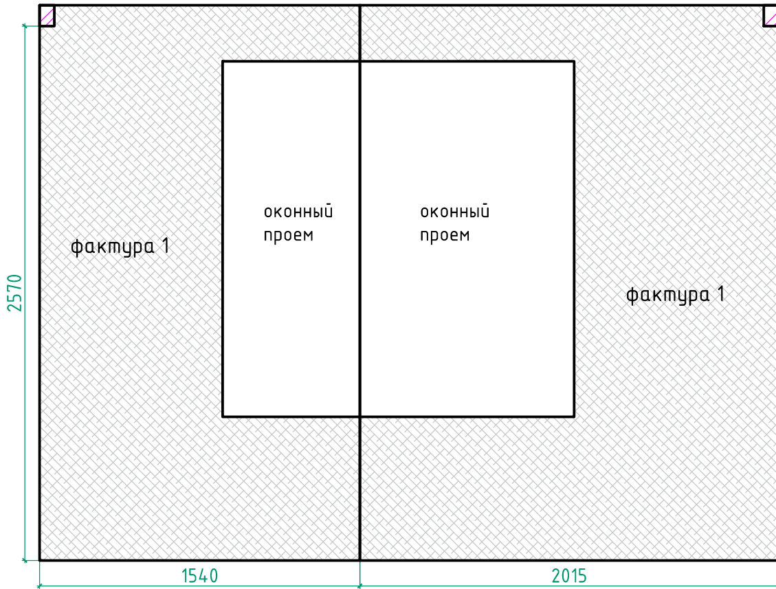
Вид Г2(кухня)
