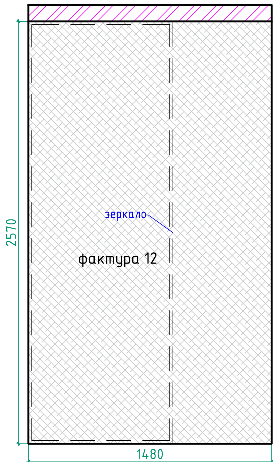
Вид E1(гардероб)
