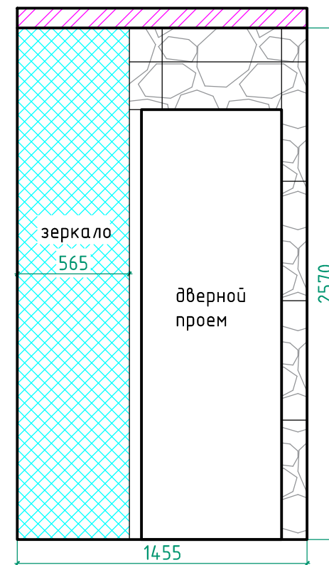
Вид Д4(Туалет)
